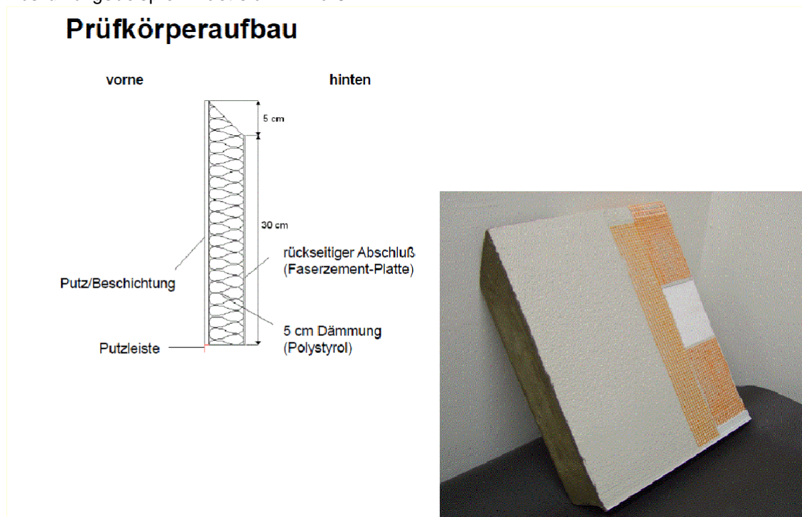
Bild 3: Schematisches Beispiel für einen geeigneten Prüfkörperaufbau.
